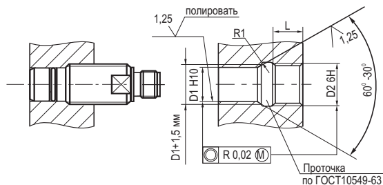
Схема монтажа
